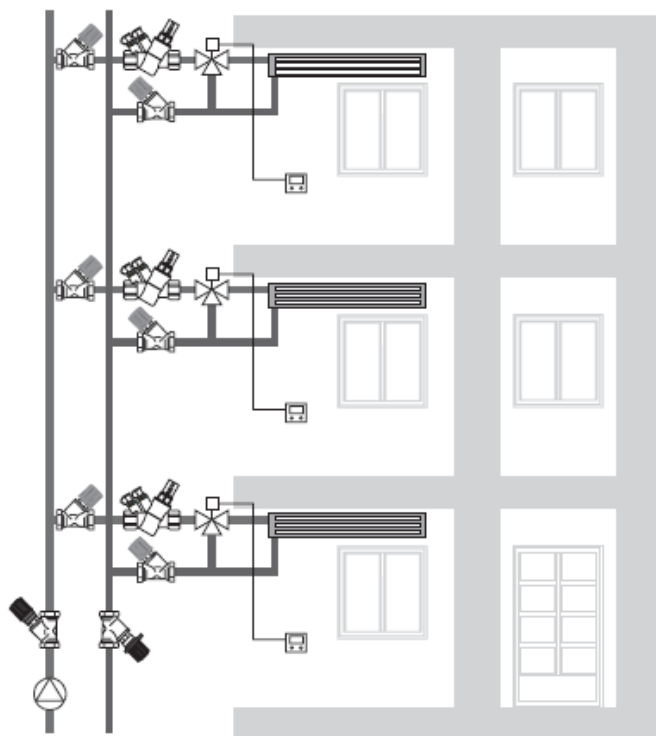
Rys. 3. Klimakonwektory z bypassem
