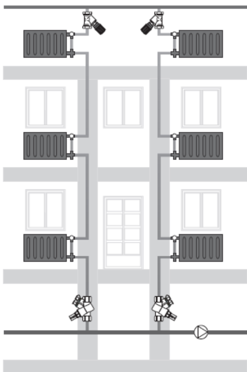
Rys. 2. Instalacja 1-rurowa
